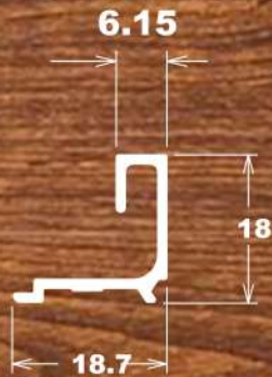
LG-027 0,149 Kg/m
