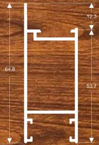
SU-245 0,672 Kg/m
