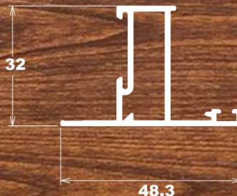
LG-091 0,151 Kg/m
