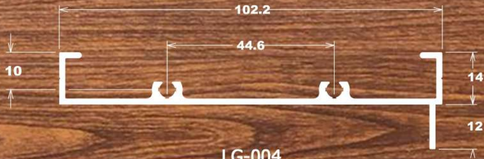
LG-004 0,757 Kg/m
