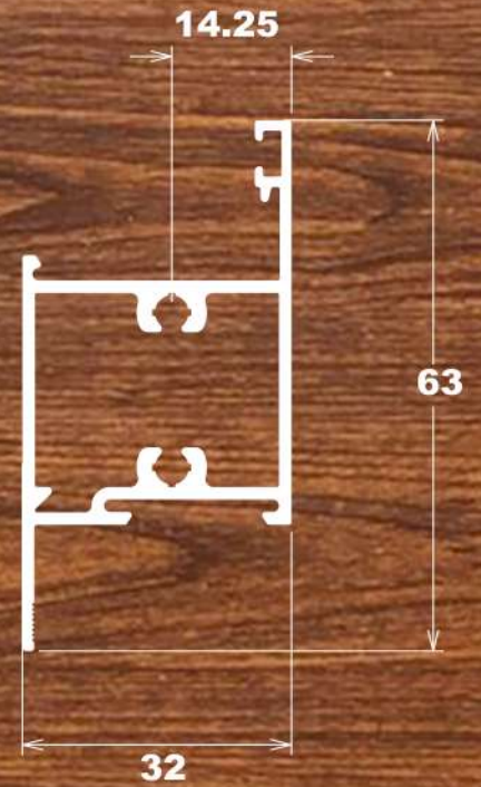
LG-076 0,765 Kg/m
