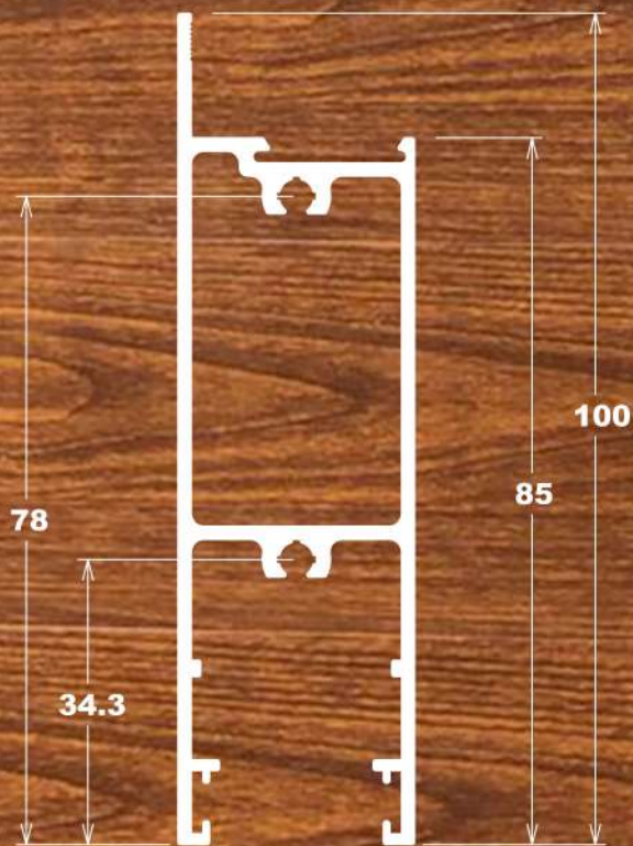
LG-007 1,229 Kg/m
