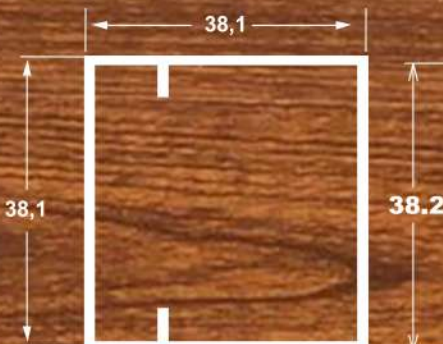
D-102 0,627 Kg/m
