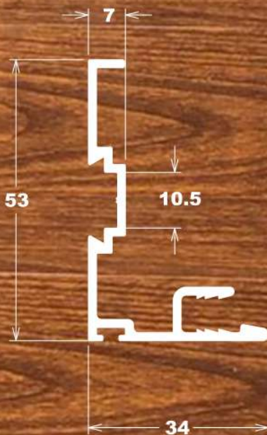
LG-023 0,551 Kg/m
