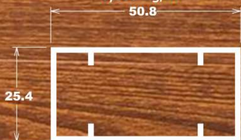
D-079 0,563 Kg/m
