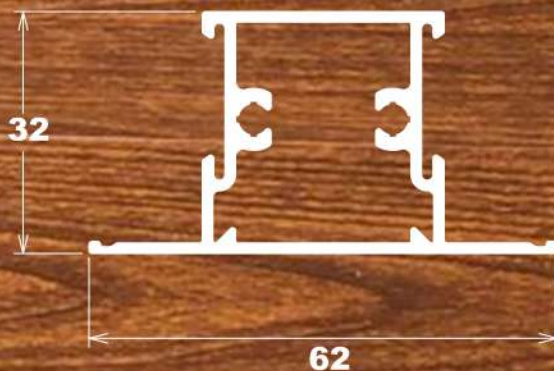
LG-079 0,770 Kg/m
