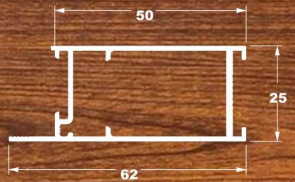
SU-245 0,672 Kg/m
