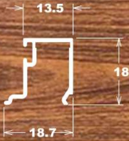
BG-057 0,170 Kg/m
