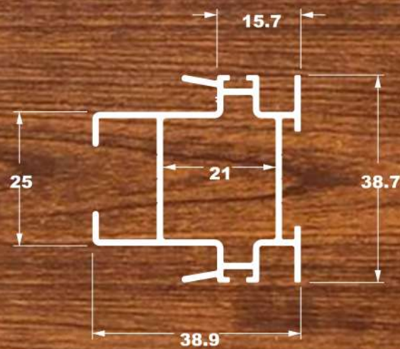
SU-057 0,631 Kg/m
