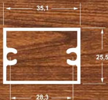
D-055 0,580 Kg/m
