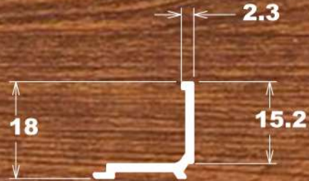
LG-015 0,147 Kg/m
