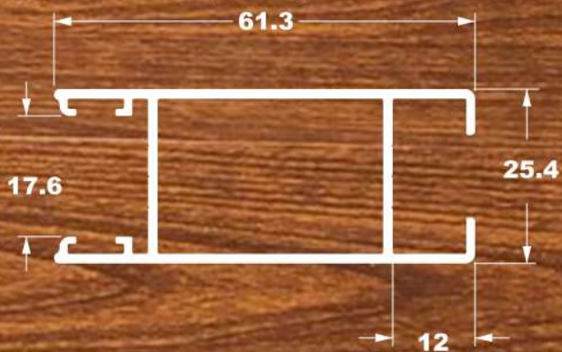
SU-238 0,714 Kg/m
