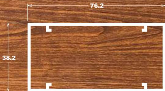
D-069 0,945 Kg/m
