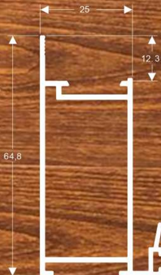
SU-242 0,742 Kg/m
