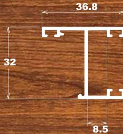
LG-068 0,405 Kg/m
