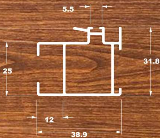
SU-056 0,539 Kg/m
