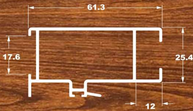
SU-239 0,783 Kg/m
