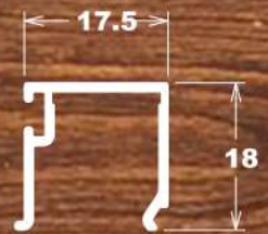
LG-059 0,169 Kg/m
