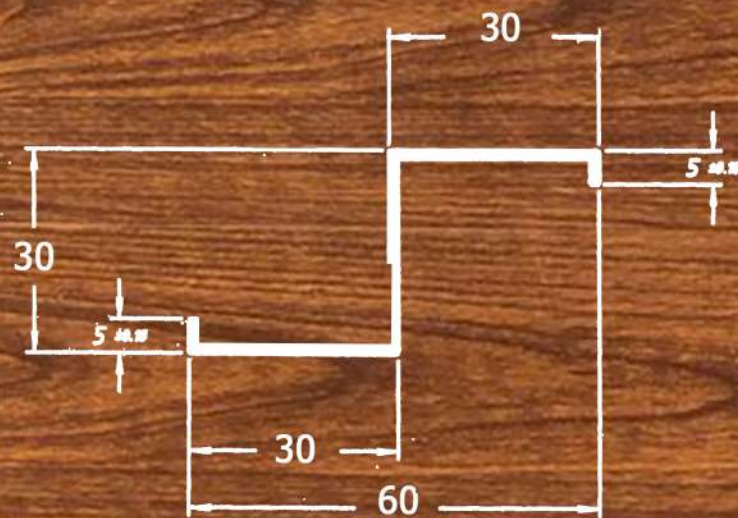
SP-001 0,327 Kg/m
