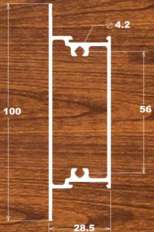
LG-022 1,064 Kg/m
