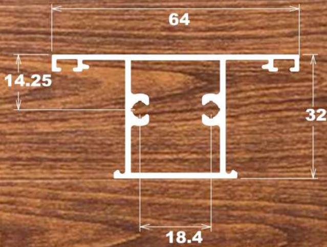
LG-074 0,760 Kg/m
