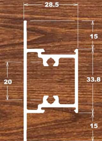
LG-055 0,759 Kg/m
