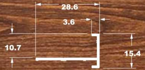
SU-100 0,157 Kg/m
