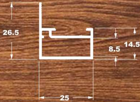
SU-276 0,169 Kg/m
